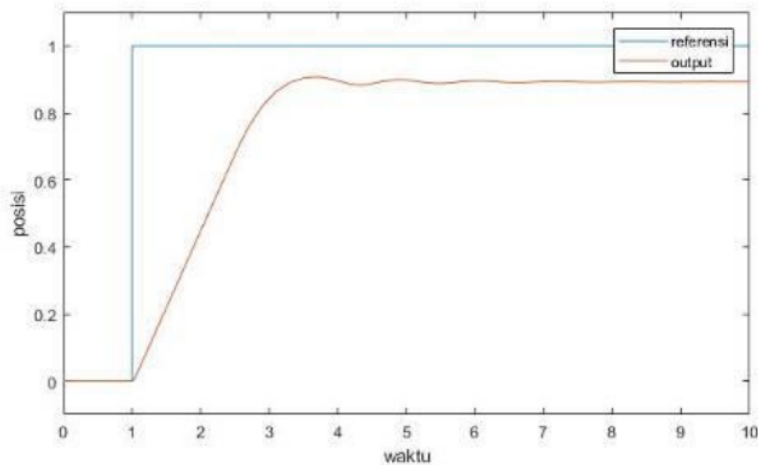
Gambar 5 Respon Sistem MSD dengan kontroler Fuzzy
