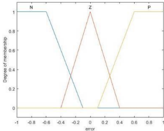
Gambar 4.a Fungsi Keanggotaan input error
