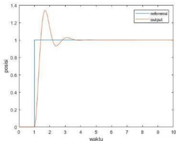
Gambar 3 Respon sistem MSD dengan kontroler PI
