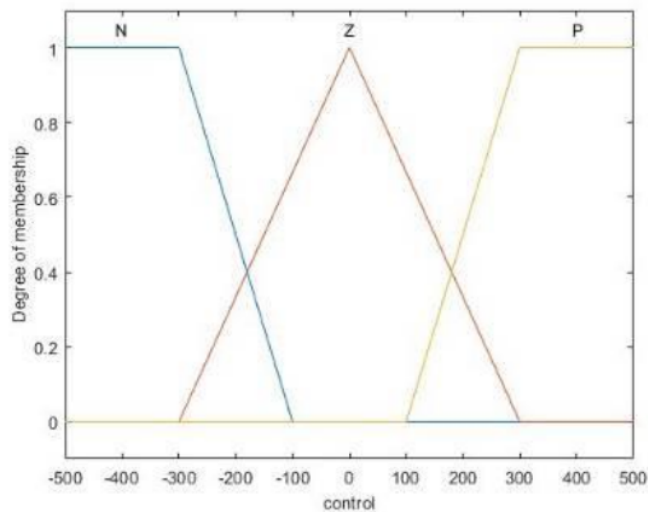
Gambar 4.c Fungsi Keanggotaan output u
