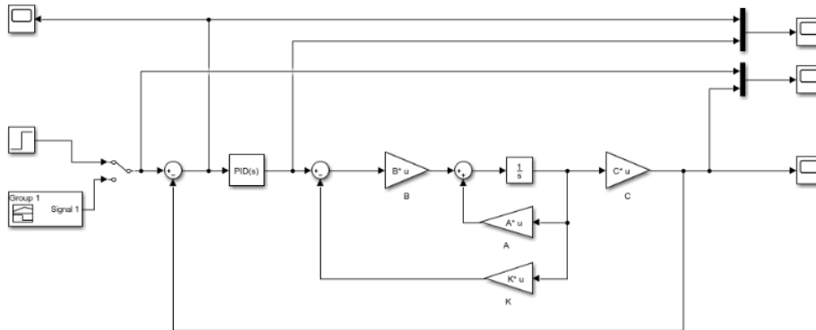
Gambar 1 Model Sistem MSD menggunakan kontroler PI
