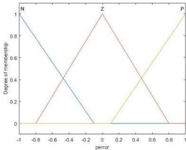
Gambar 4.b Fungsi Keanggotaan input perror
