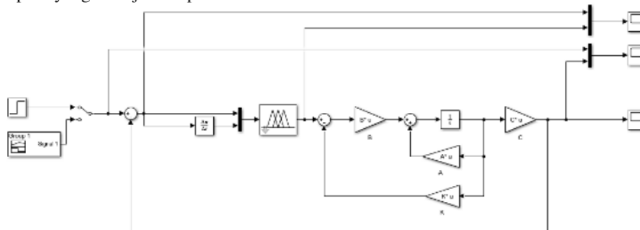
Gambar 2 Model Sistem MSD menggunakan kontroler Fuzzy-Mamdani
